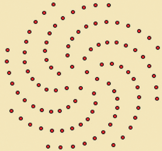
FERMAT SPIRAL
