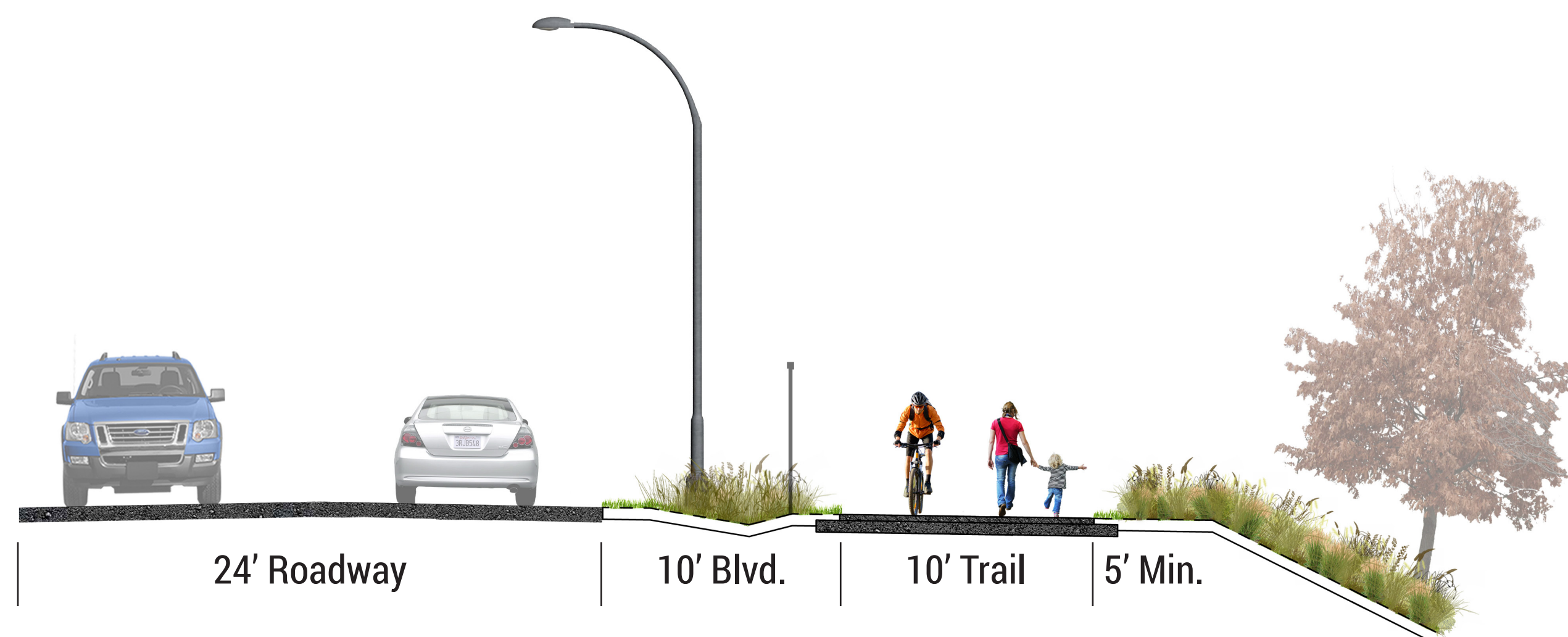
Eaton Street - Typ. Section E2
