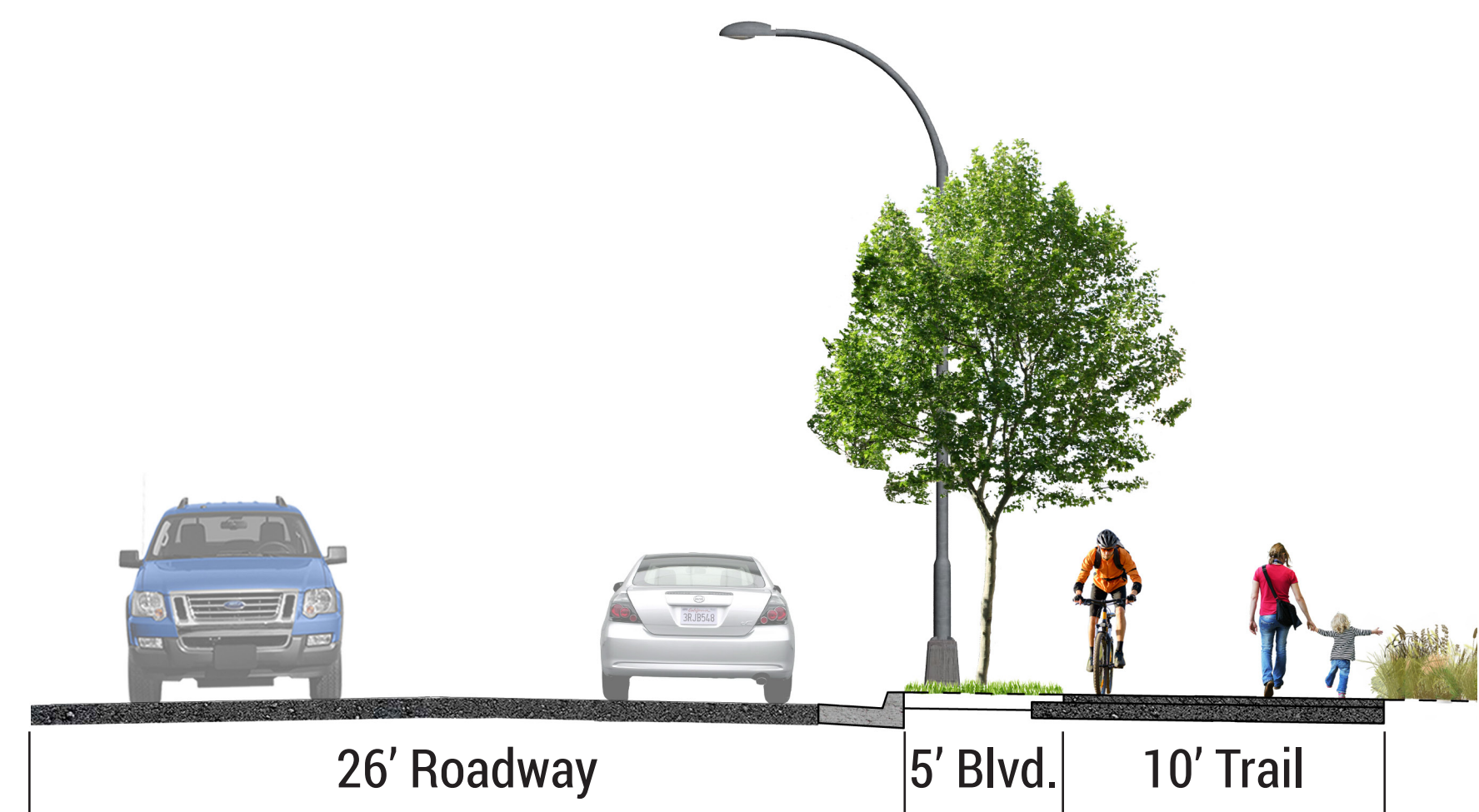
Eaton Street - Typ. Section E1
