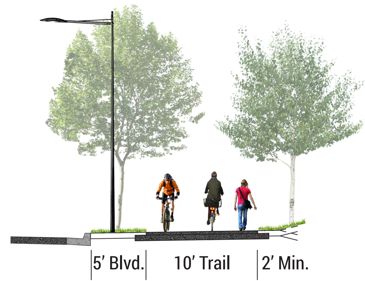
Frontage Road - Typ. Section F1
